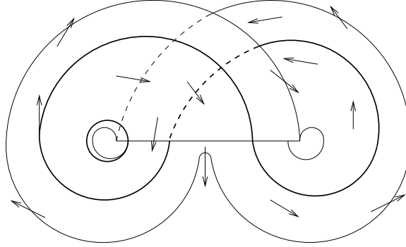
Fig. 3. The Lorenz template
