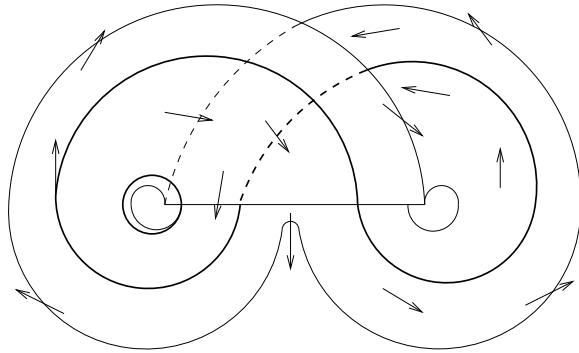
Fig. 3. The Lorenz template
